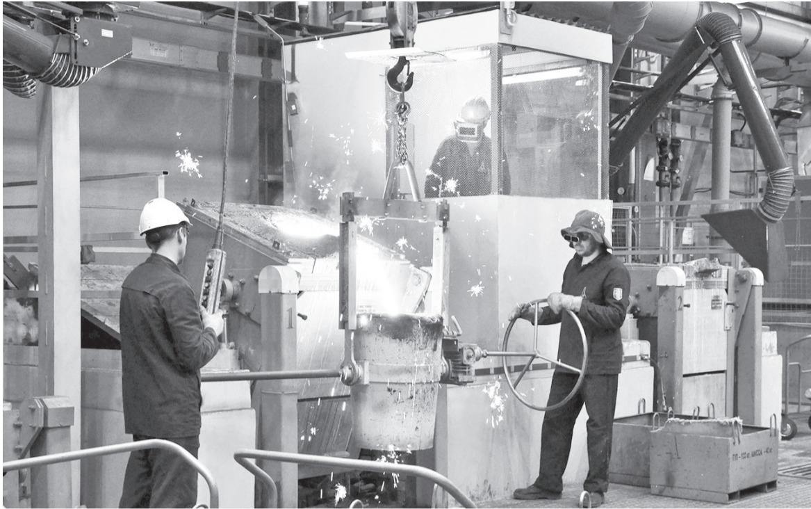
Процесс заливки литья в форму
